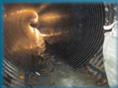
Le PECQ – Tubage de la buse ARMCO Diamètre 3 250 m sur 280 m
